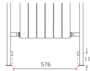
Yüz tarafı mesafeleri (mm)
