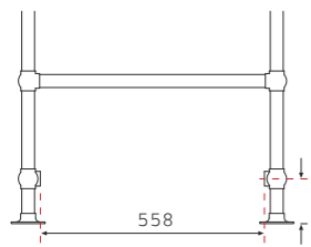
Yüz tarafı mesafeleri (mm)
