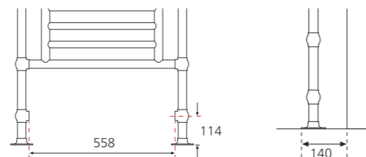
Yüz tarafı mesafeleri (mm) Duvardan dışarı taşma (mm)
