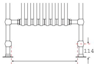
Boru eksenleri arası mesafe (mm)
