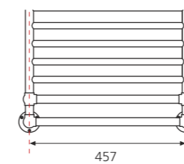
Boru eksenleri arası mesafe (mm)
