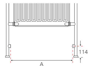
Boru eksenleri arası mesafe (mm)
